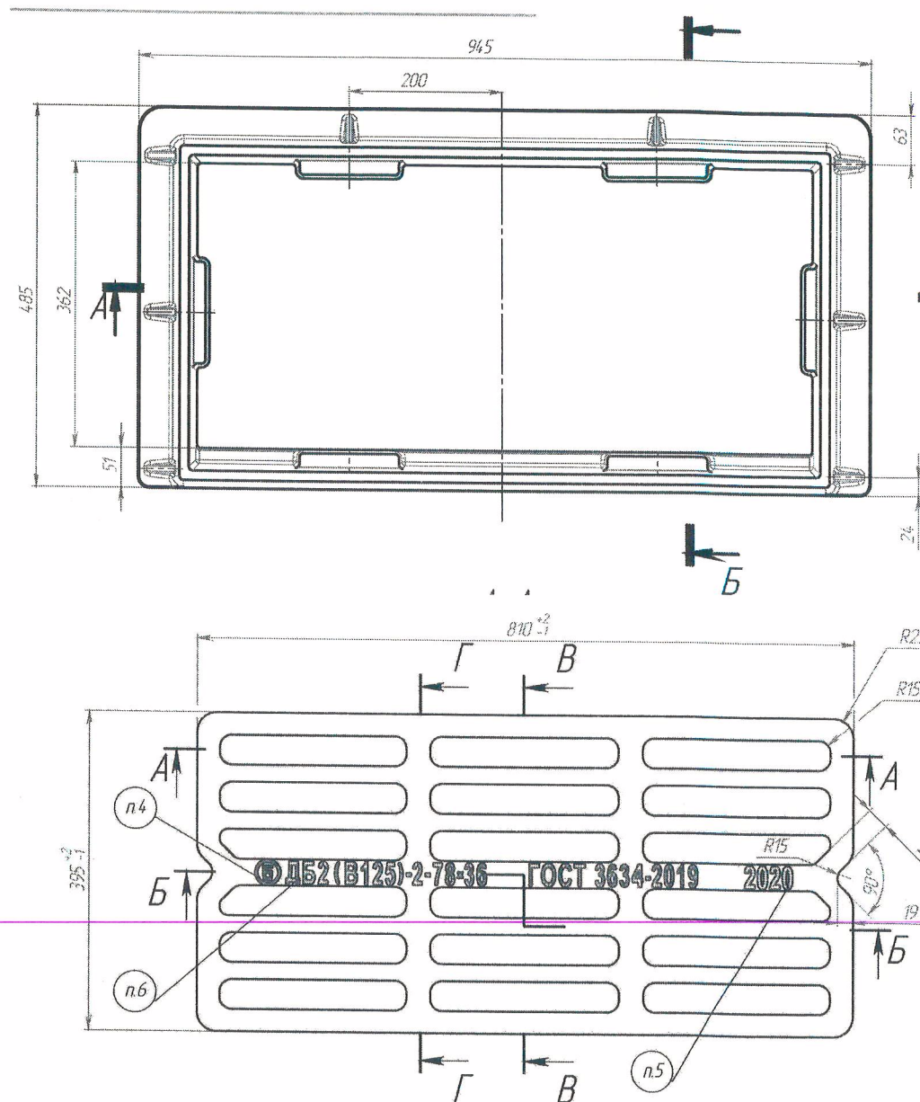
Люк чугунный прямоугольного дождеприемника типа «ДБ2» (В125) 2-78 * 36 Г О С Т 3634-2019.
