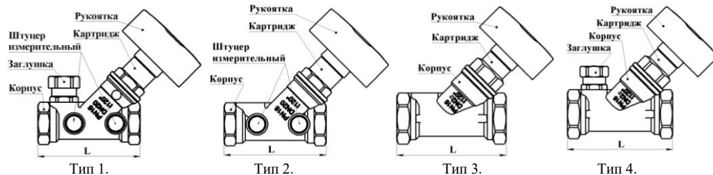
Рисунок 1. Клапан балансировочный ручной STAD.BY.
