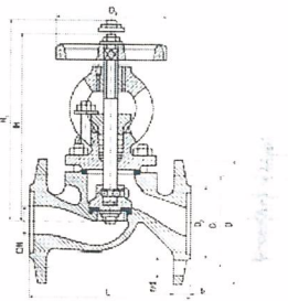
ЧЕРТЕЖ ОБЩЕГО ВИДА
