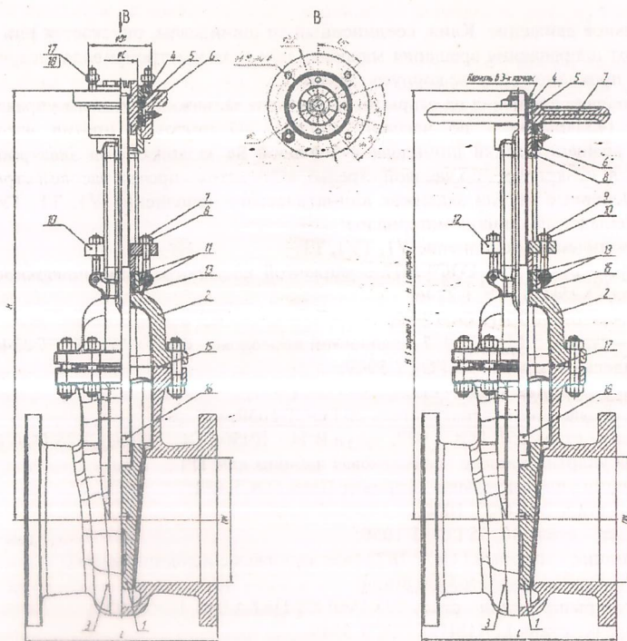
Рисунок 1. Задвижка клиновая с выдвижным шпинделем под электропривод (редуктор)
