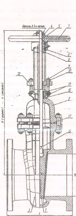
Рисунок 2. Задвижка клиновая с выдвижным шпинделем с ручным приводом
